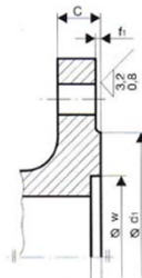
Typ G: Wypust na uszczelkę o przekroju kołowym – O-ring
