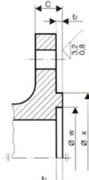
Typ C: Występ
